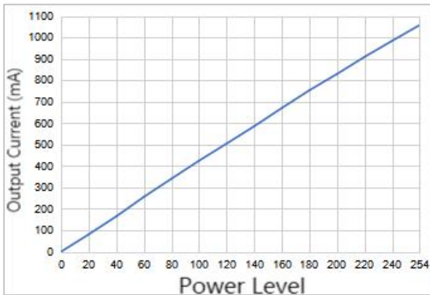
Linear dimming
